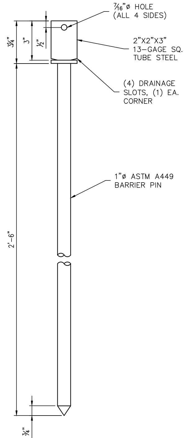
ELEVATION VIEW SCALE: 2" = 1'-0"
